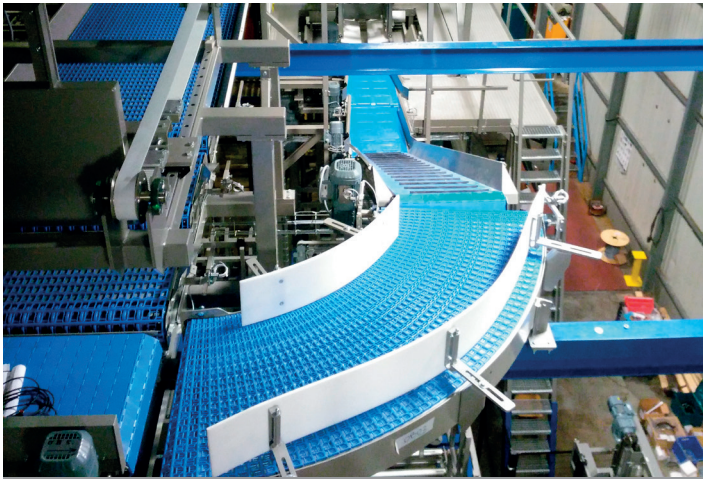
Hoekband / opvoerband
