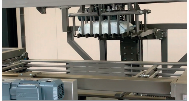
Grijperkop met zakkenlift
